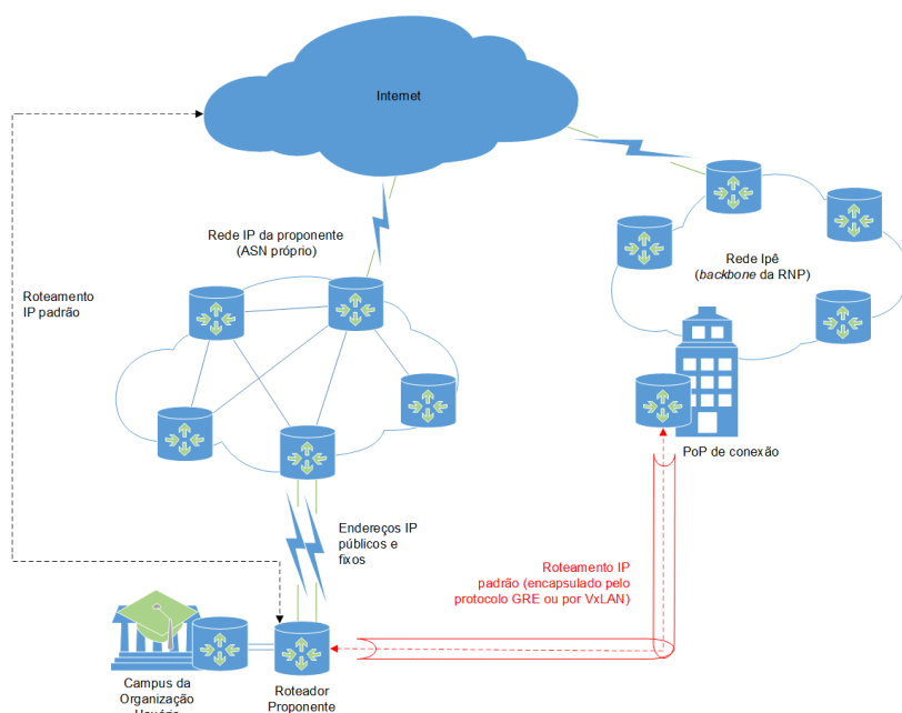
Figura 3 Porta IP com túnel GRE.
