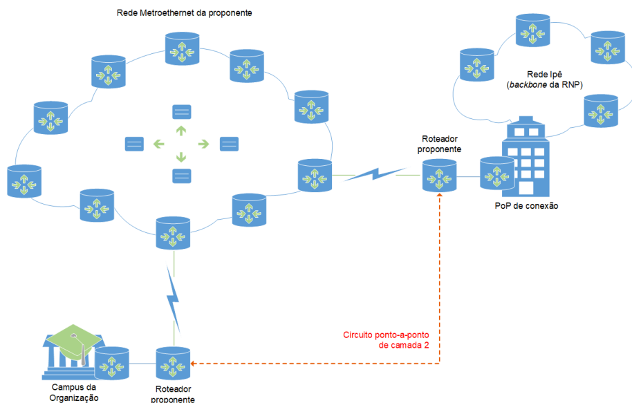
Figura 1 Circuito Metroethernet.
