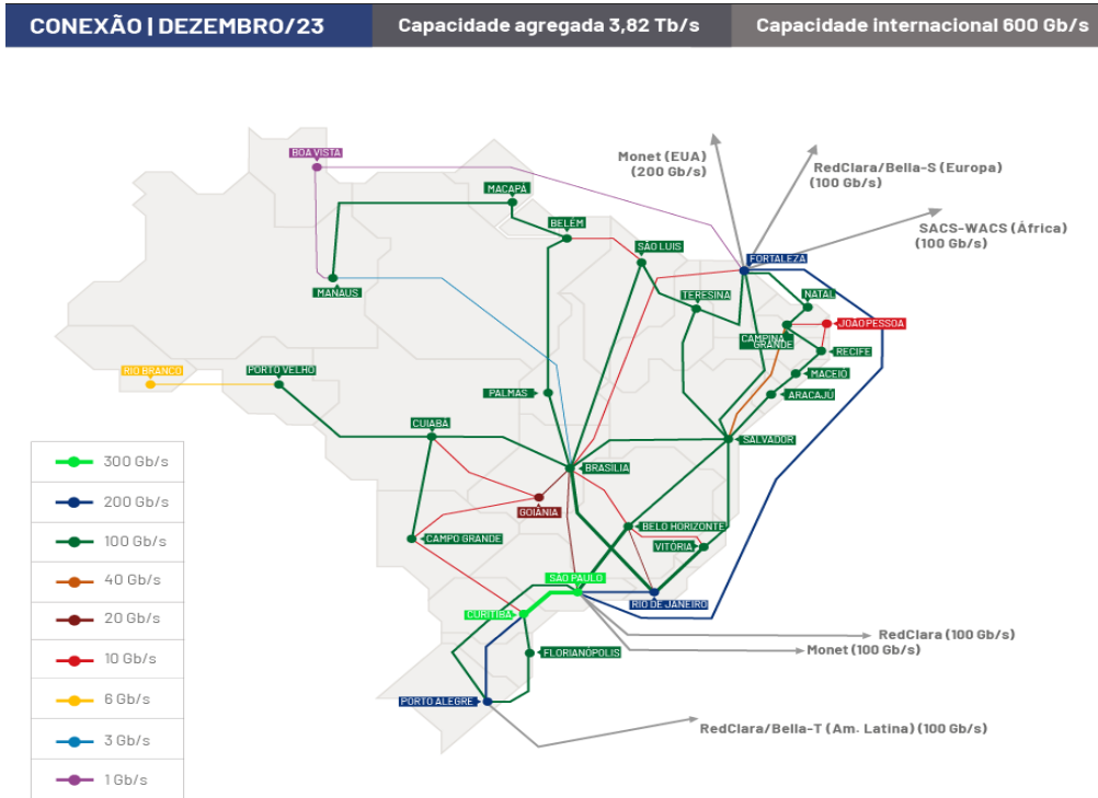
Figura 1: Rede Ipê, o backbone nacional da RNP
