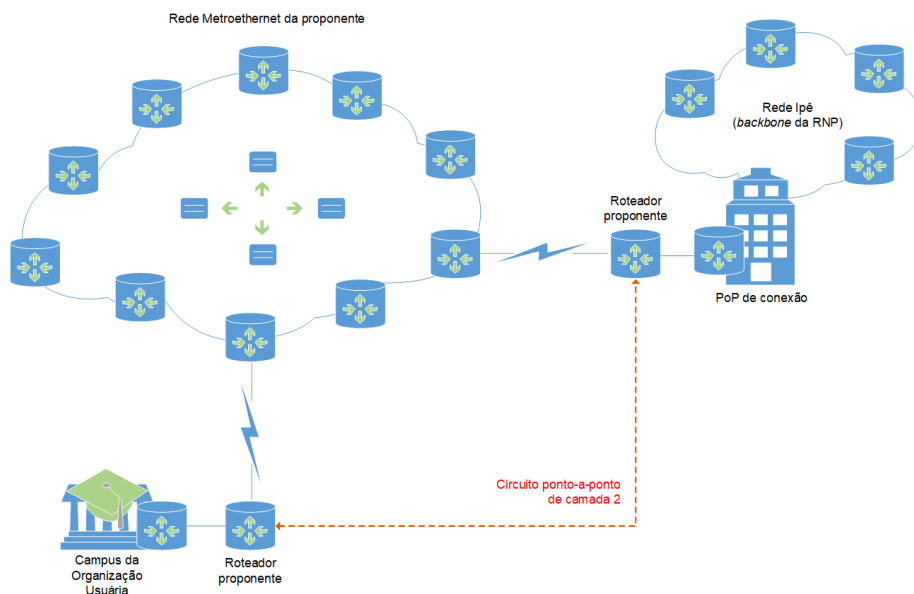
Figura 1 Circuito Metroethernet.
